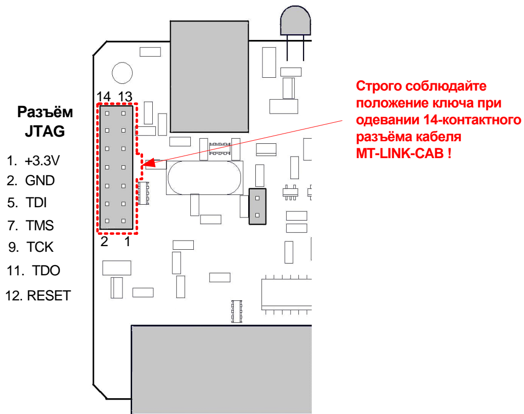
Рис. 5-2. Разъём JTAG
