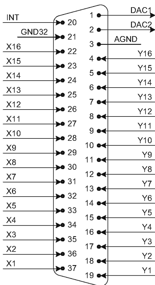
Рис. 5-1: Разъем ANALOG.
