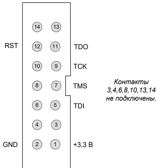
Рис. 5-5. Разъём JTAG
