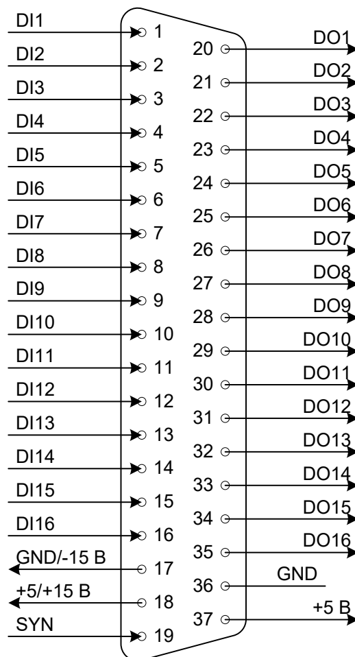
Рис. 5-2: Разъем DIGITAL
