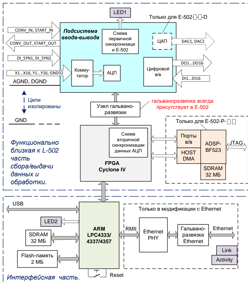
Рис. 3-5. Функциональная схема
