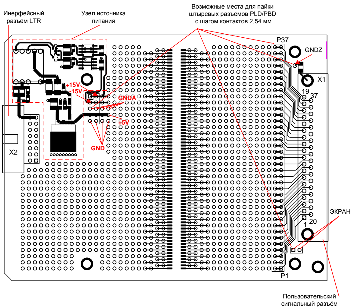
Рис. 1 Внешний вид печатной платы модуля LTR00
