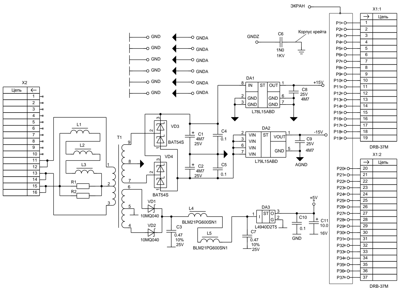
Рис. 5 Схема электрическая LTR00-01
