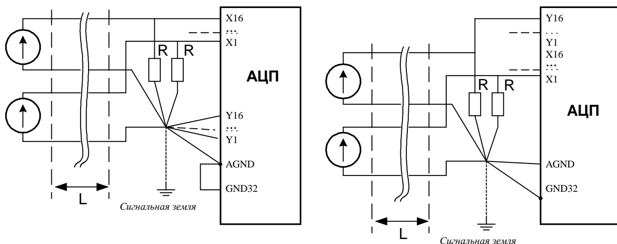
РИС 1. Особый случай подключения сигналов “по току”: дифференциальный режим (слева), однофазный (с общей землёй, справа).
